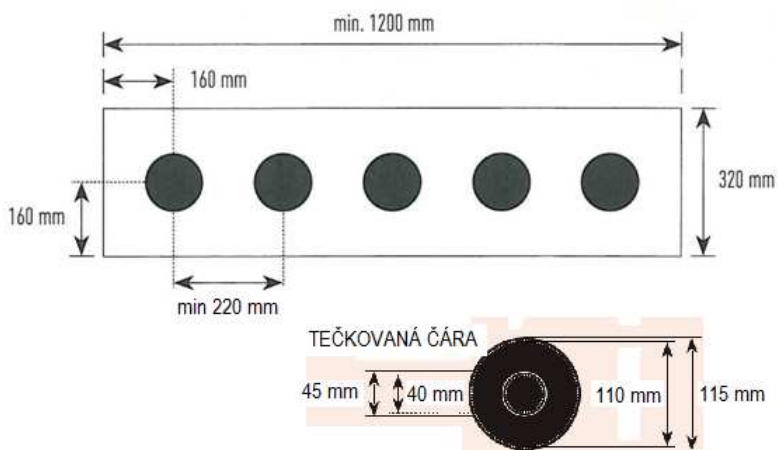
Obr. 3 Normované rozměry papírových terčů
