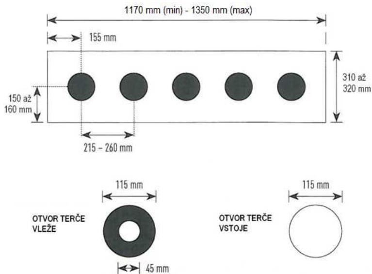
Obr. 3 Normované rozměry papírových terčů
