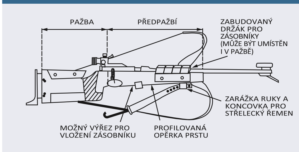
OBRÁZEK 1 BIATLONOVÁ ZBRAŇ
