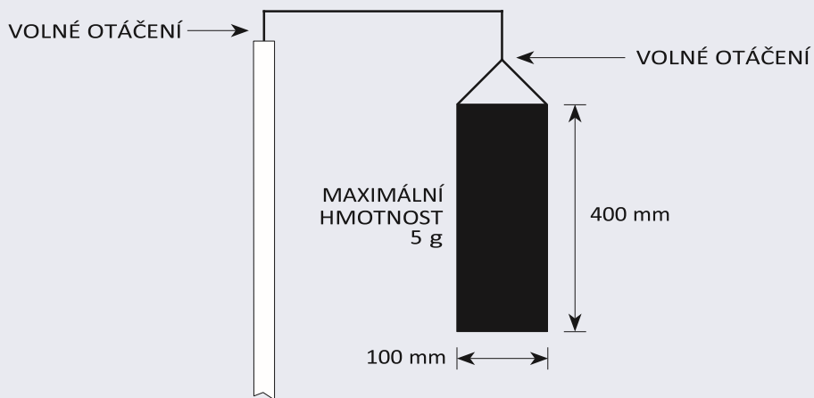
OBRÁZEK 2 NORMOVANÉ ROZMĚRY KOVOVÝCH TERČŮ
